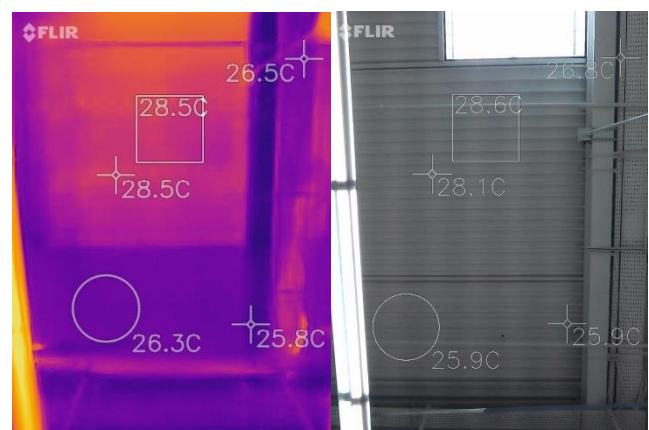
Thermographie IR du plafond sous la zone non peinte et zone peinte avec Cool Roof France
