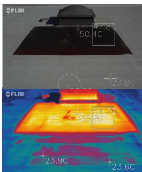
Thermographie IR du revêtement de surface extérieur de la zone non peinte et zone peinte avec Cool Roof France
